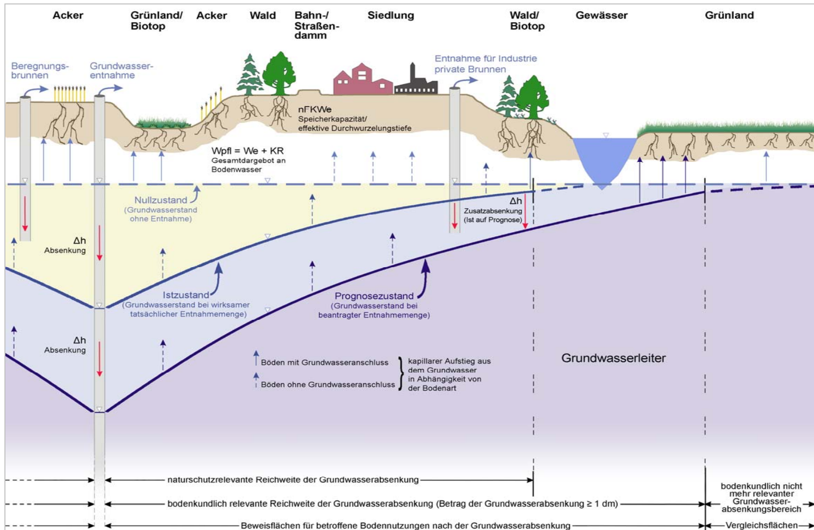
Abb. 4: Schematische Darstellung der Auswirkungen einer Grundwasserentnahme: Betrag und Reichweite der Absenkung – Nullzustand, Istzustand und Prognosezustand (Entwurf: F. Raissi).
